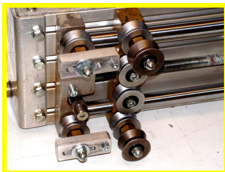
SOSTENTATORI PER L'USO NELLA SALDATURA DEI BULBI
