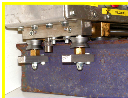
SOSTENTATORI PER L'USO NELLA SALDATURA DEI BULBI
