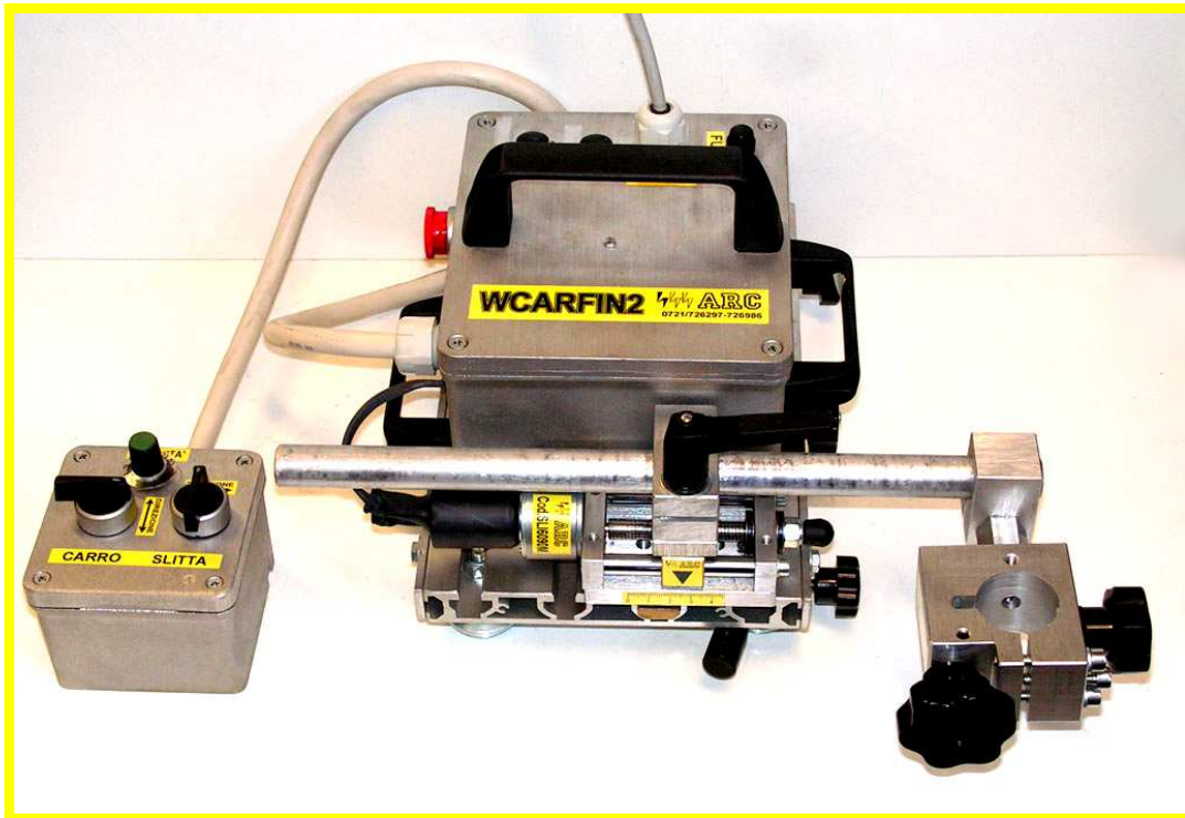
VISTA LATERALE CON SLITTA MOTORIZZATA, CON SUPPORTO PORTACANNELLO E TASTIERINO PER COMANDI A DISTANZA.
